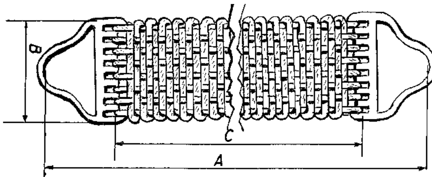
n°860 BROEKSTROPPIEN - ELINGUES à SACS in Manilatouw of staaldraadtouw
